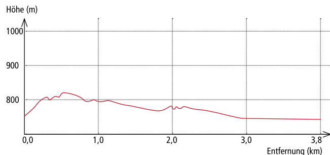
Abbildung 1: Geländeschnitt „Hammersbach-Tour“ (Variante a)
